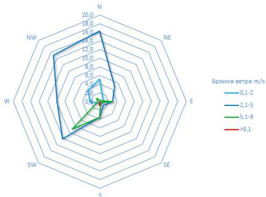
Графикон 1. Графички приказ Руже ветрова за период 2011-2020. године - Метеоролошка станица Кукавица
